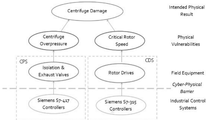
Attaque Stuxnet sur les centrifugeuses iraniennes
